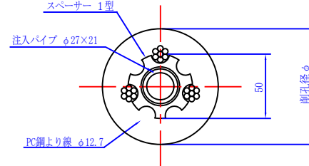
B-B断面図 S=1/3
