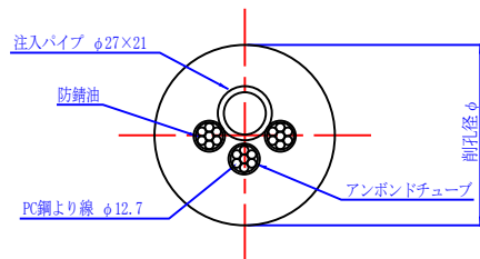
A-A断面図 S=1/3
