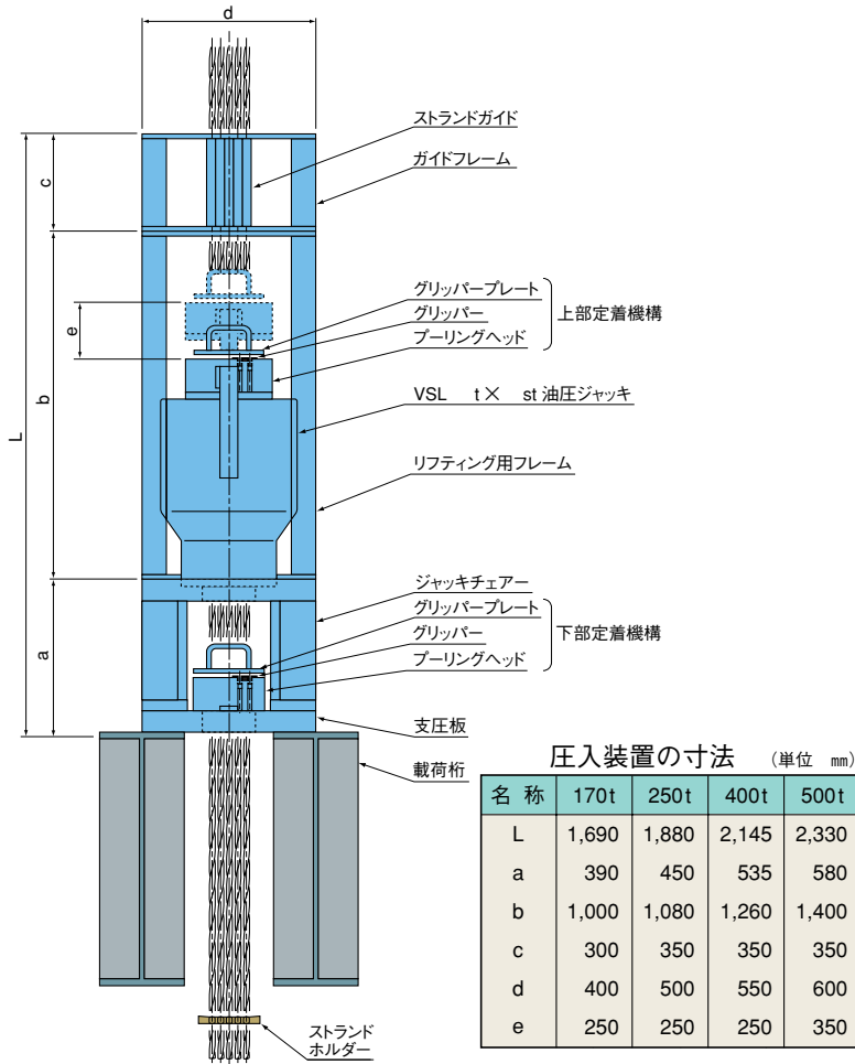
圧入装置図
