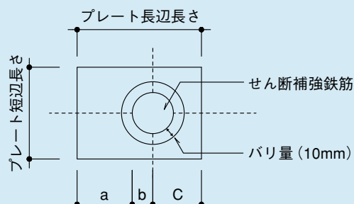
プレート寸法と鉄筋径の関係
