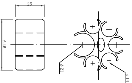
スプーサー S=1/1 #60
