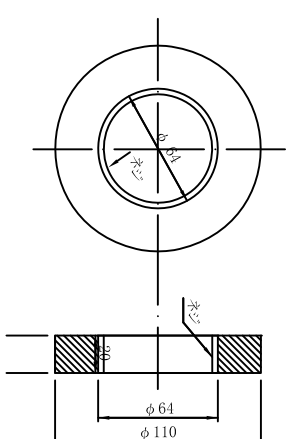
ジョイントプレート S=1/2 (E5-4タイプ)
