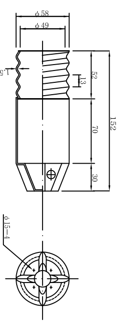
エンドキャップ S=1/2 #60
