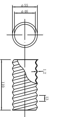
ジョイントスリーブ S=1/2 #60
