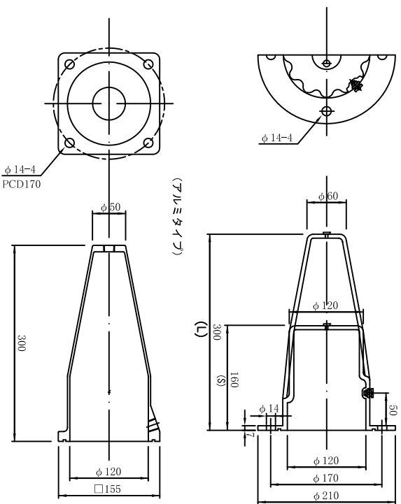
ヘッドキャップ S=1/4 (樹脂タイプ) (L, S) (E5-4タイプ)
