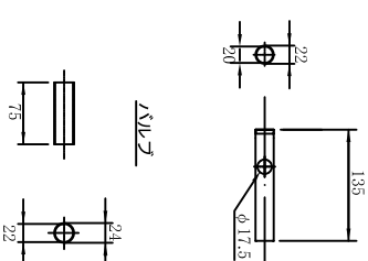
スリーパルク S=1/5 スリーブ
