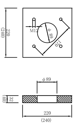
支圧板 S=1/5 (溶融亜鉛メッキ) (E5-4タイプ) コンクリート強度 \sigma_{cp}=20\text{N}/\text{mm}^2 (15N/ \text{mm}^2 )
